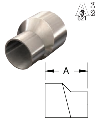
BPE Table DT-4.1.3-1 ASME BPE 2019
