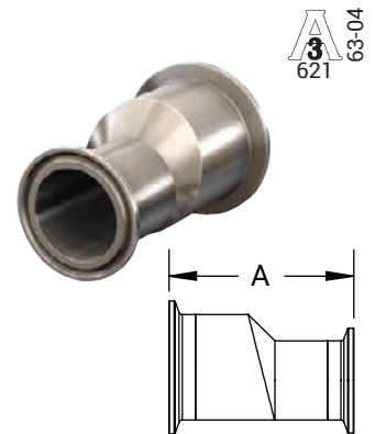
BPE Table DT-4.1.3-3 ASME BPE 2019
