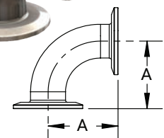
BPE Table DT-4.1.1-3 ASME BPE 2019
