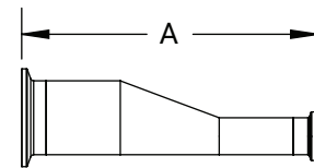
BPE Table DT-4.1.3-3(a)
